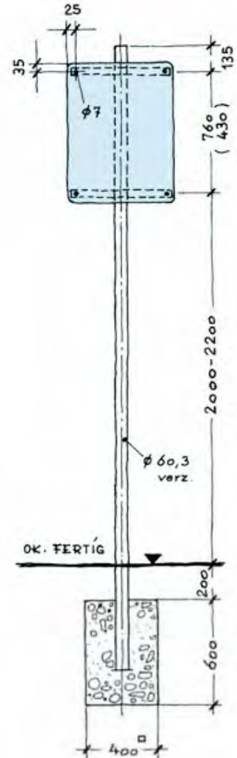
Abb. 1 Montagebeispiel am Rohrpfeiler (Angaben in mm)
