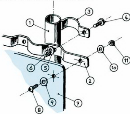
Abb. 2 Montage der Schilderhalterung H 380 und H 600
